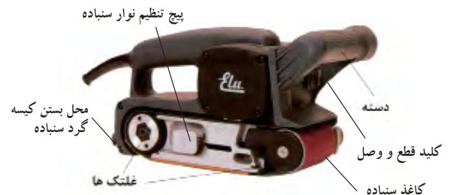
شکل ۷-۵- امزای مهم و کاربردی دستگاه سنباده نواری.
