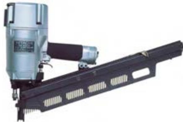
شکل ۸-۱۸- میخ‌کوب، برای اتصال چوب‌های ضمیمه.
