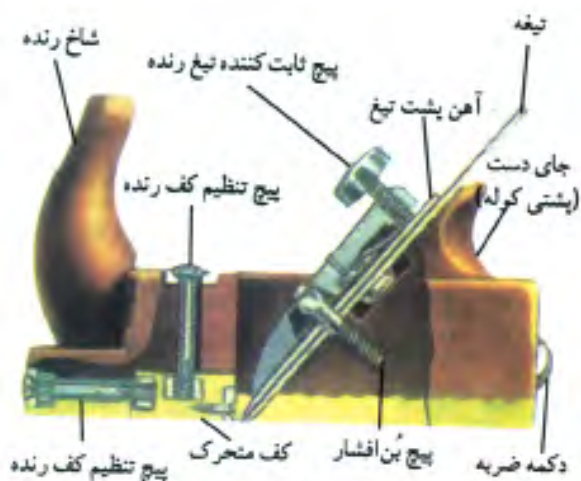
شکل ۲-۲- رنده‌ی دو تیغ چوبی.
