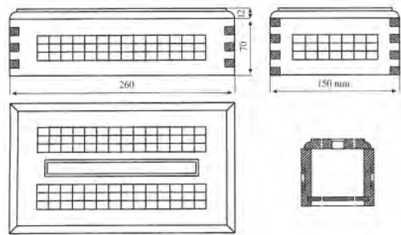
شکل ۹-۷۳ - نقشه‌ی سه‌نمای جعبه‌ی دستمال کاغذی به همراه برش عرضی.
