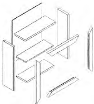
شکل ۸۲-۱۲- تصویر مجسم انفجاری جعبه‌ی کمک‌های اولیه.
