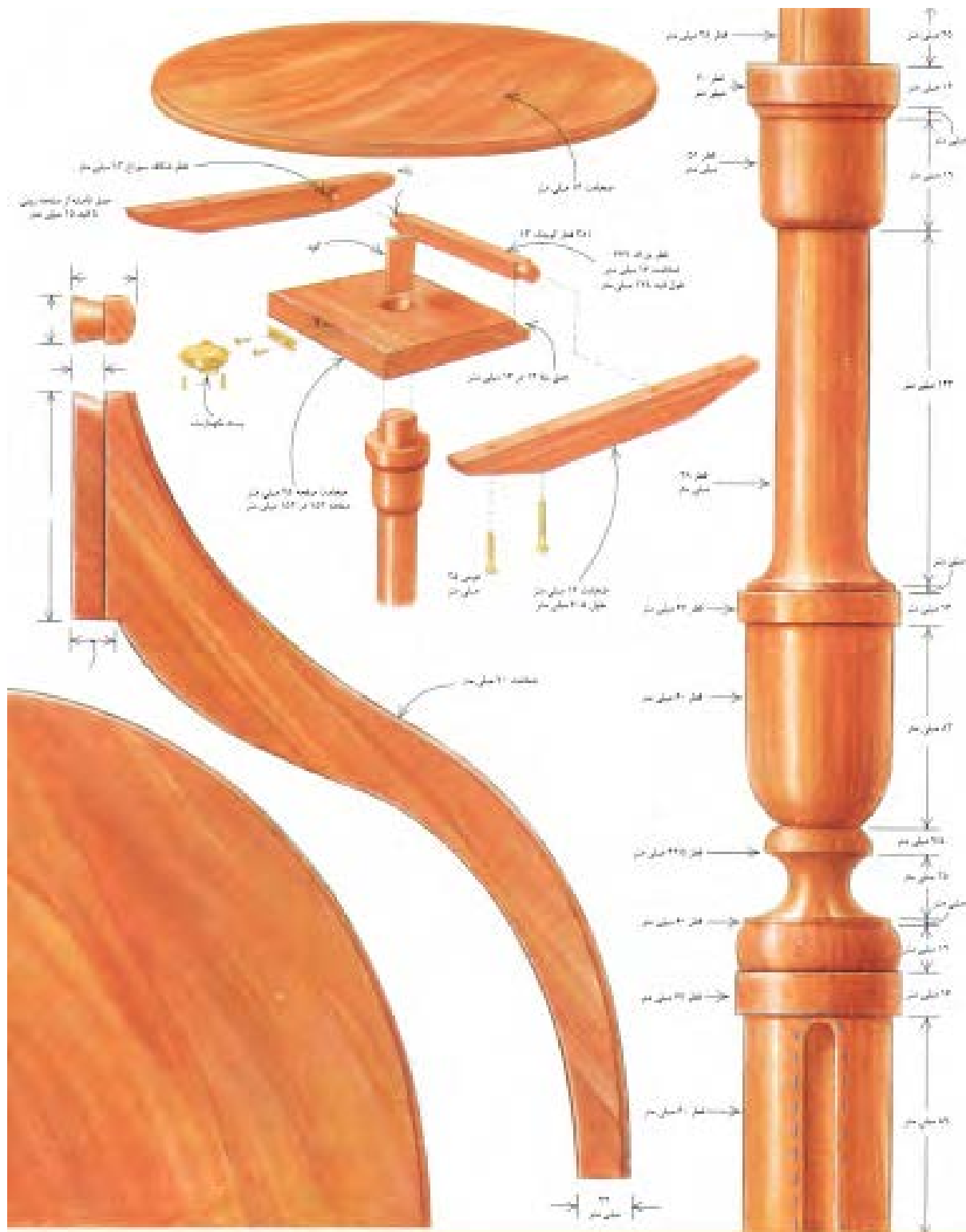
نوعه: پایه در شکل نشان داده شده ایمان واقعی ندارد. برای ساخت آن باید تصویر فوق را بزرگتر نموده و سپس از آن فتوکپی بگیرید و به عنوان شابلون آن را ببرید.
