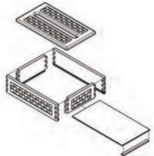
شکل ۹-۵۶. نقشه‌ی انفجاری جعبه‌ی دستمال کاغذی.
