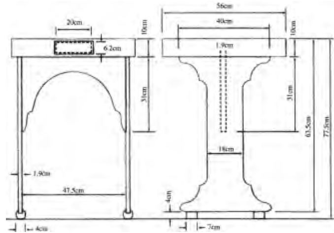
شکل ۱۵۹-۱۲- دو نمای اصلی میز شطرنج.
