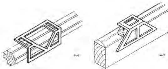
شکل ۷-۱- الف) شابلن دو طرف فارسی، ب) شابلن یک طرف فارسی و یک طرف ۹۰ درجه.
