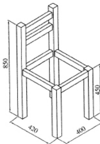
شکل ۹-۱۱۲- تصویر ایزومتریک صندلی.
