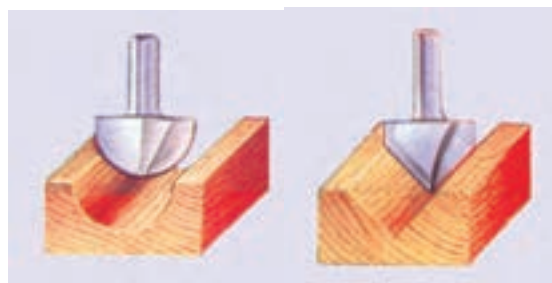
شکل ۱۰-۹- نمونه‌هایی از ابزارهایی که با اورفرز ایجاد می‌شود.
