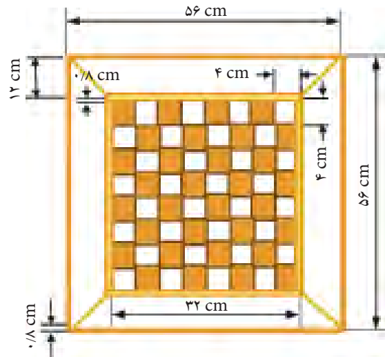
شکل ۱۶۰-۱۲- صفحه‌ی رویی میز شطرنج.
